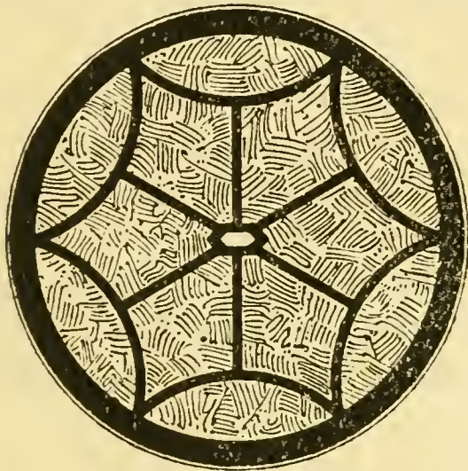
FIG. 61. Tomb on the Via Salaria (diameter 31 m.). Plan.
